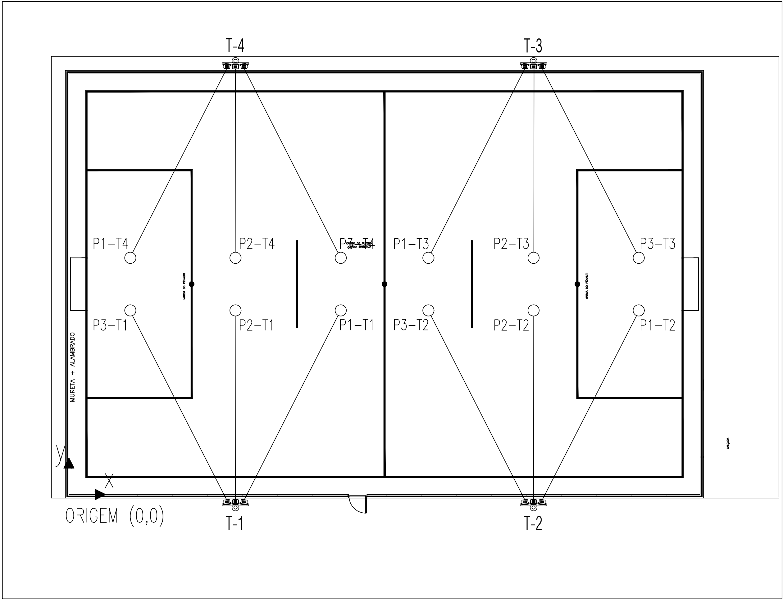
PLANTA BAIXA - FOCALIZAÇÃO DOS PROJETORES SEM ESCALA DEFINIDA
